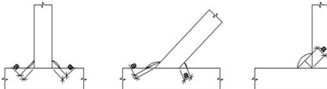
Účinná výška kútových zvarov
