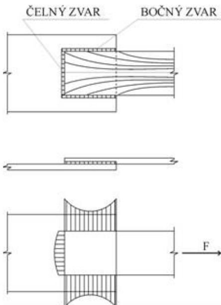
Rozdelenie napätí v čelných a kútových zvaroch
