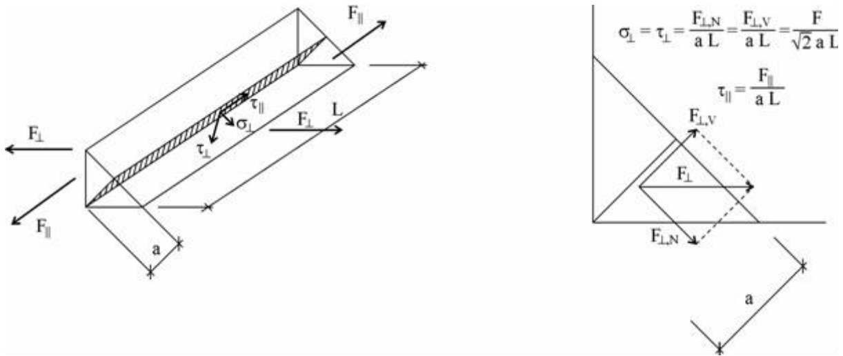
Zložky vnútorných síl vo zvaru a im prislúchajúce napätie
